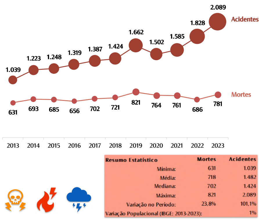
Gráfico 40 - Total de acidentes de origem elétrica – série histórica 2013-2023
