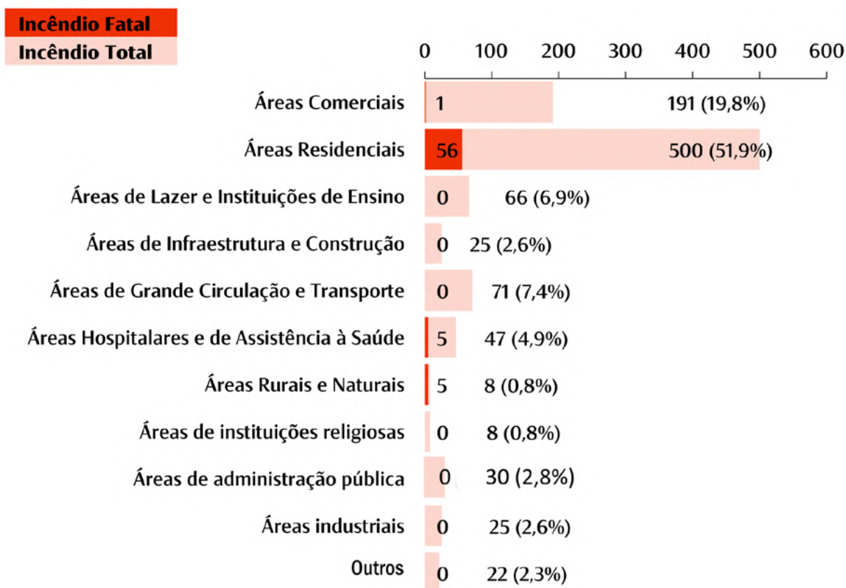
Gráfico 27 - Número de incêndios de origem elétrica por local de ocorrência em 2023
