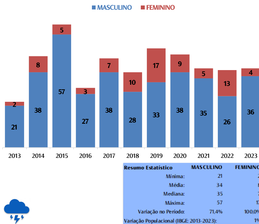
Gráfico 51 - Número de mortes decorrentes de descargas atmosféricas, por gênero – Série histórica 2013-2023
