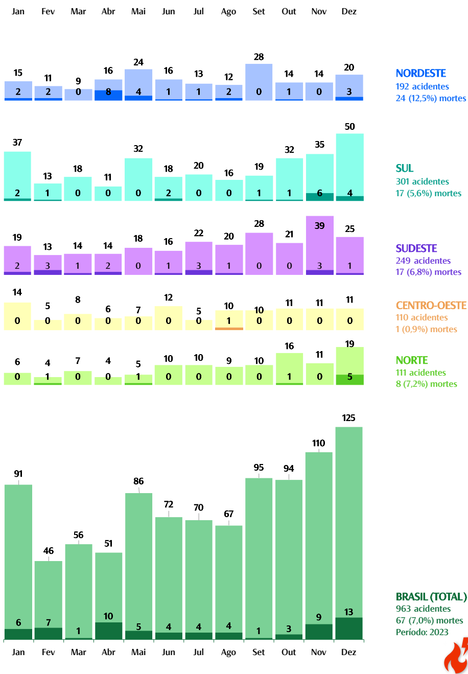
Gráfico 26 - Número de incêndios de origem elétrica por região e mês em 2023
