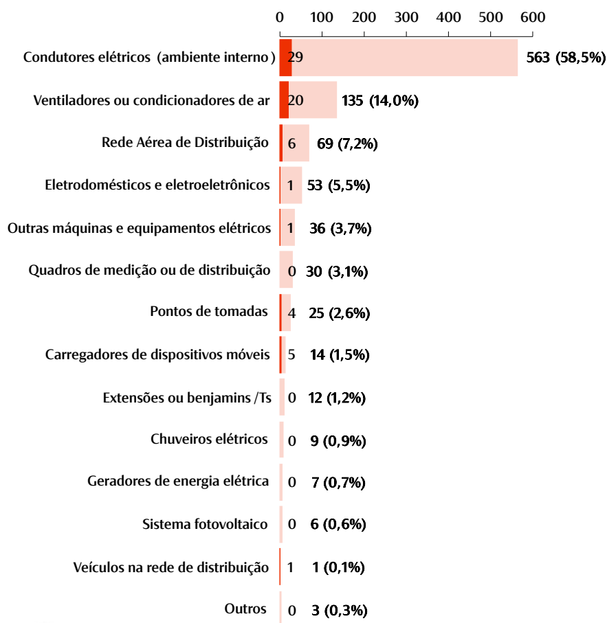
Gráfico 28 - Número de incêndios de origem elétrica por tipo de equipamento em 2023
