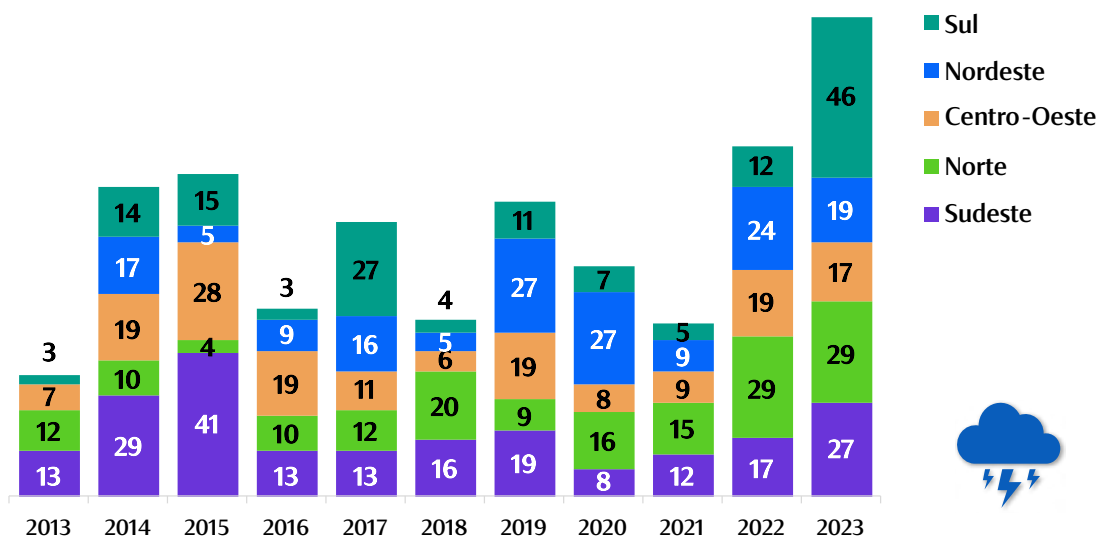
Gráfico 52 - Número de mortes decorrentes de descargas atmosféricas, por região – Série histórica 2013-2023
